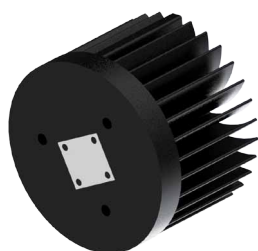
Thermal interface
