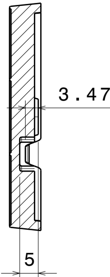
Section view B-B Scale: 1:1
